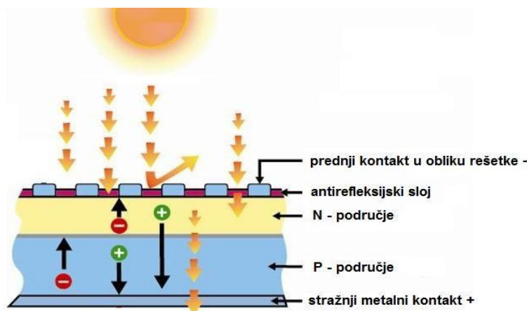
Структура фотонапонске ћелије
